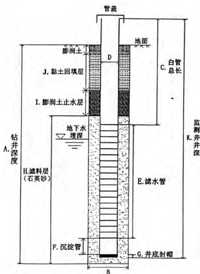
图 4.1-8 监测井剖面示意图
