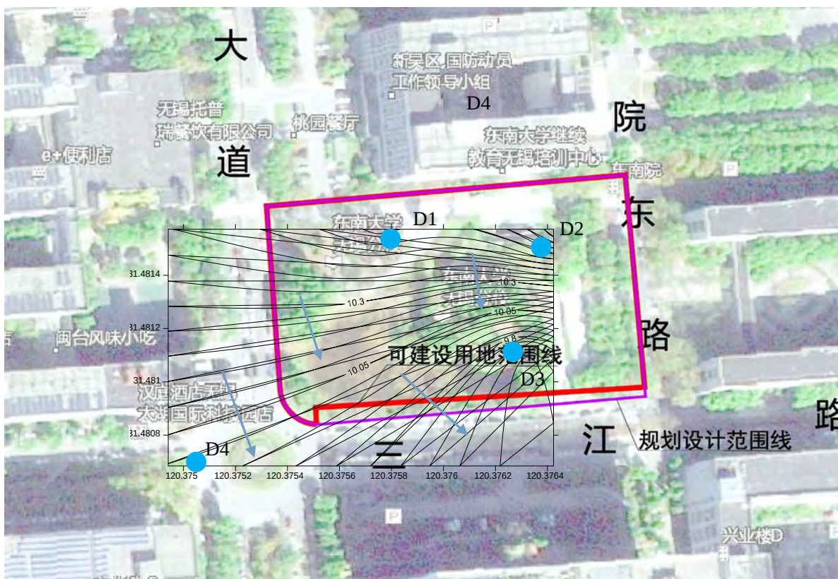
图 4.2-1 地下水流场图
