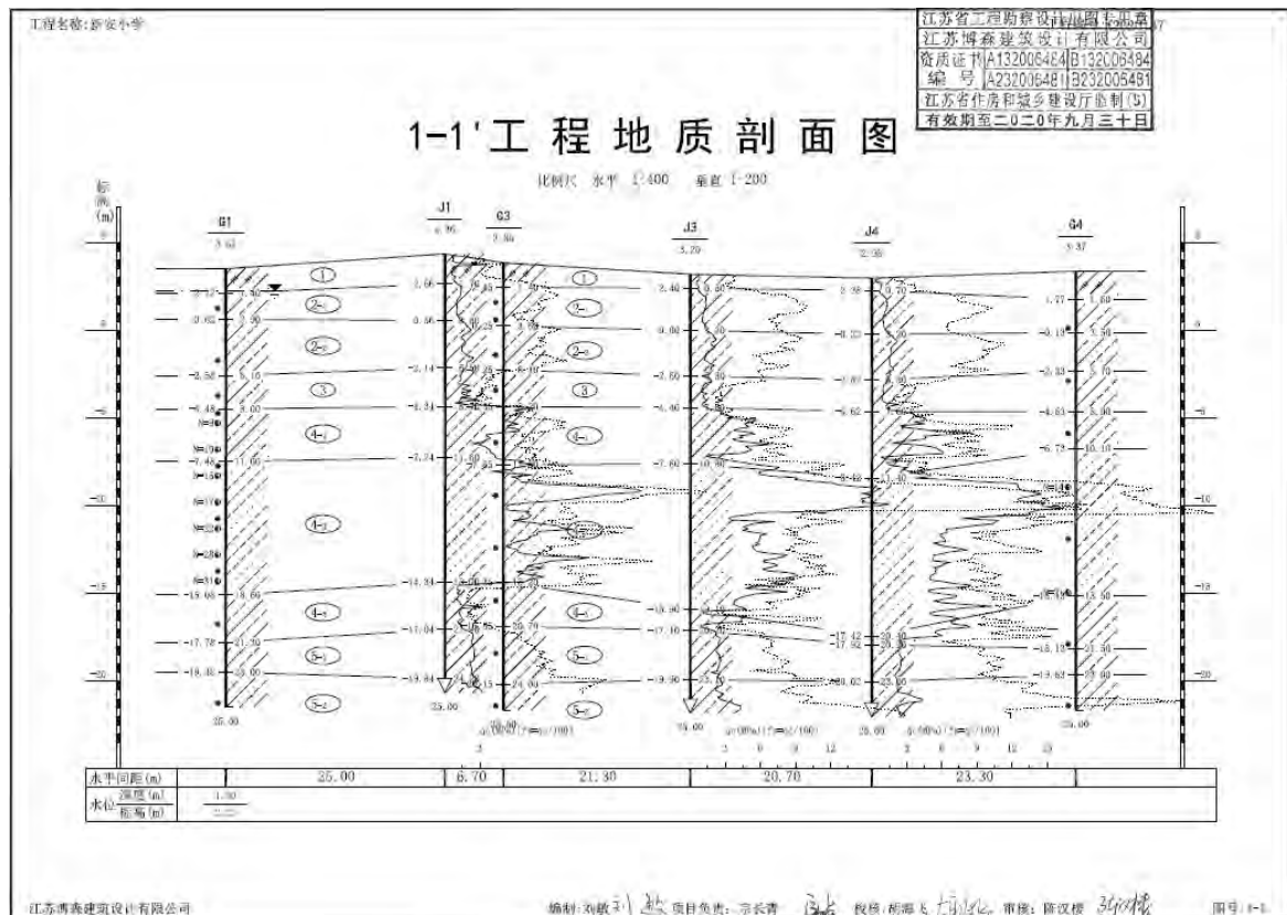
图 2.3-1 工程地质剖面图
