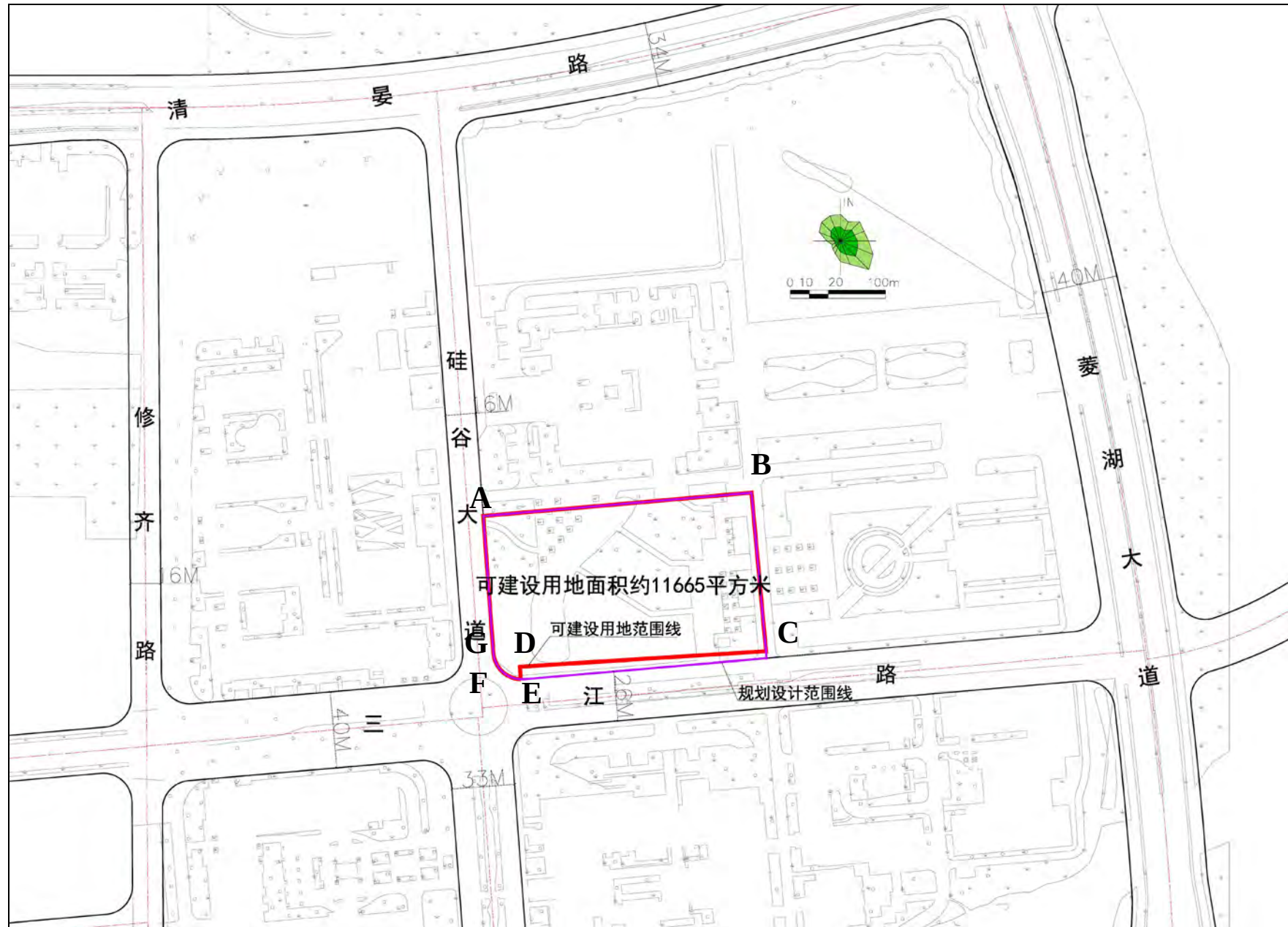
图 1.3-1 荷花池游园及配套设施工程项目范围图
