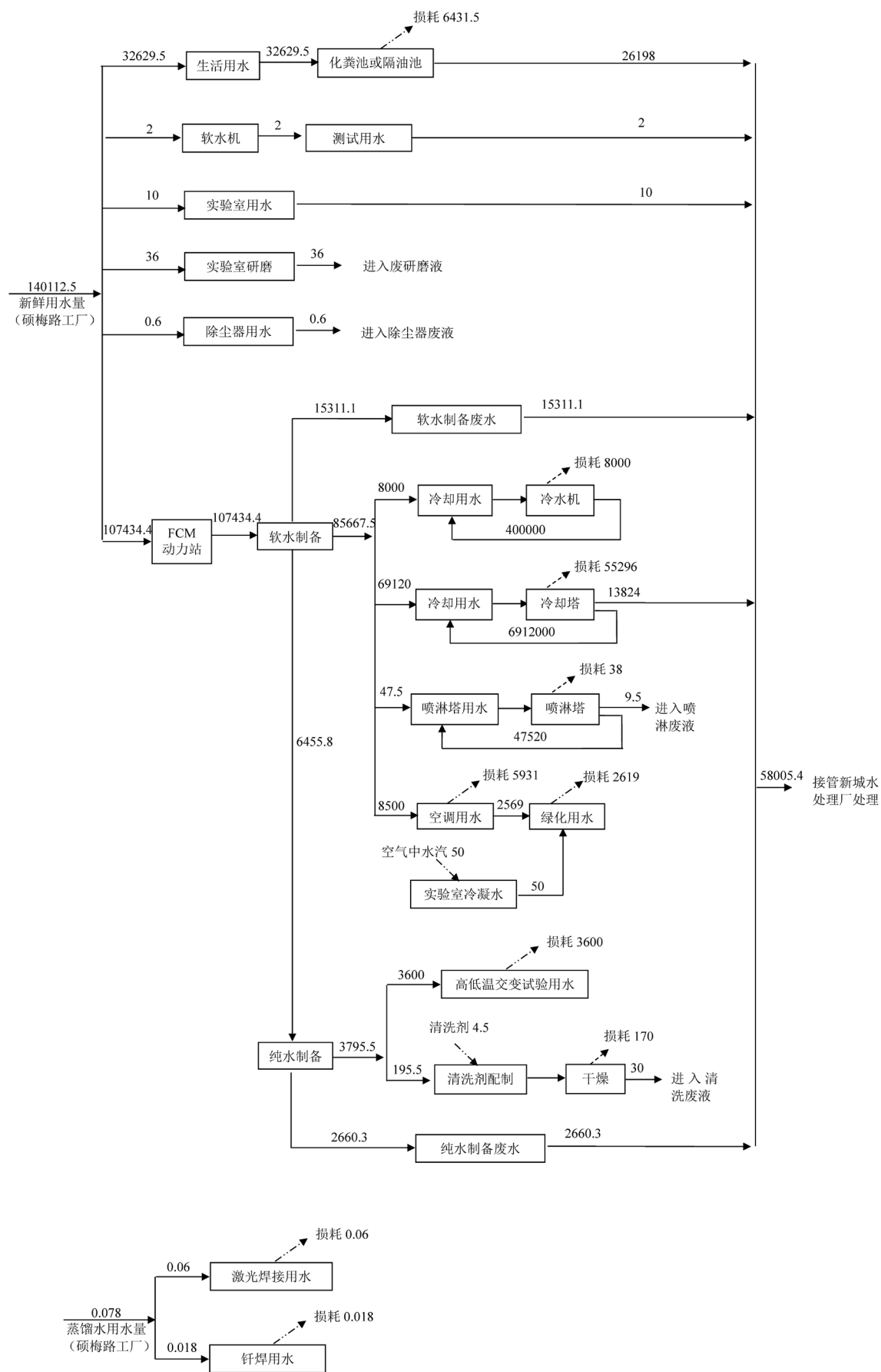
图2-2 全厂水(汽)平衡图 (单位:吨/年)
