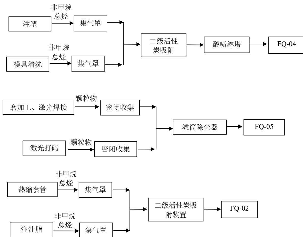
图4-2 本项目废气污染治理方案示意图
