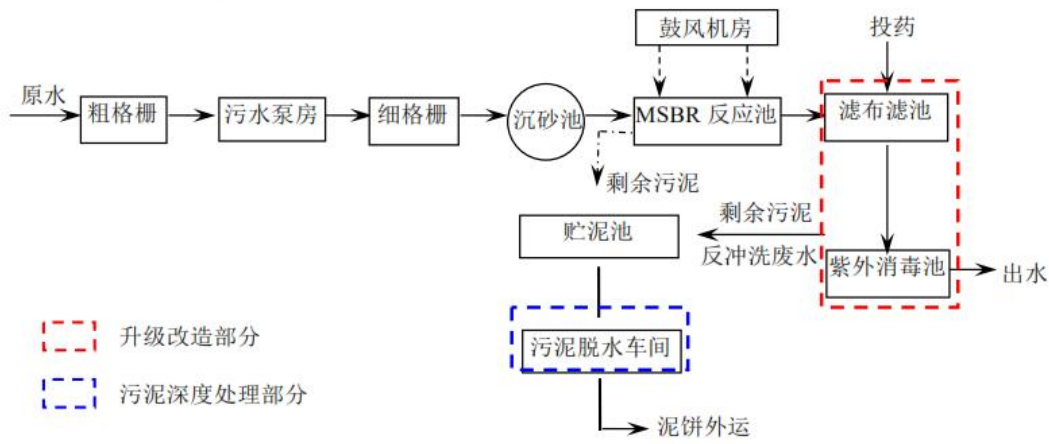
图4-1 四期工程污水处理工艺流程图
