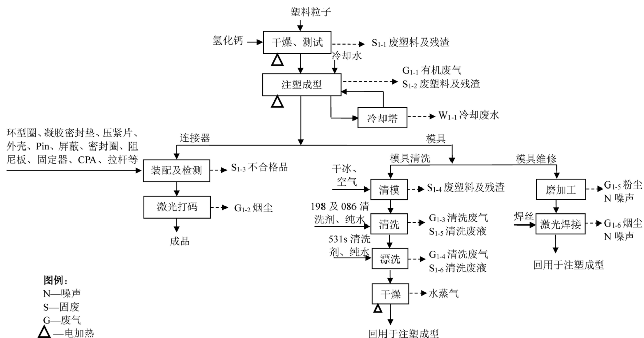
图2-3 高压连接器、低压连接器工艺流程及产污环节图
