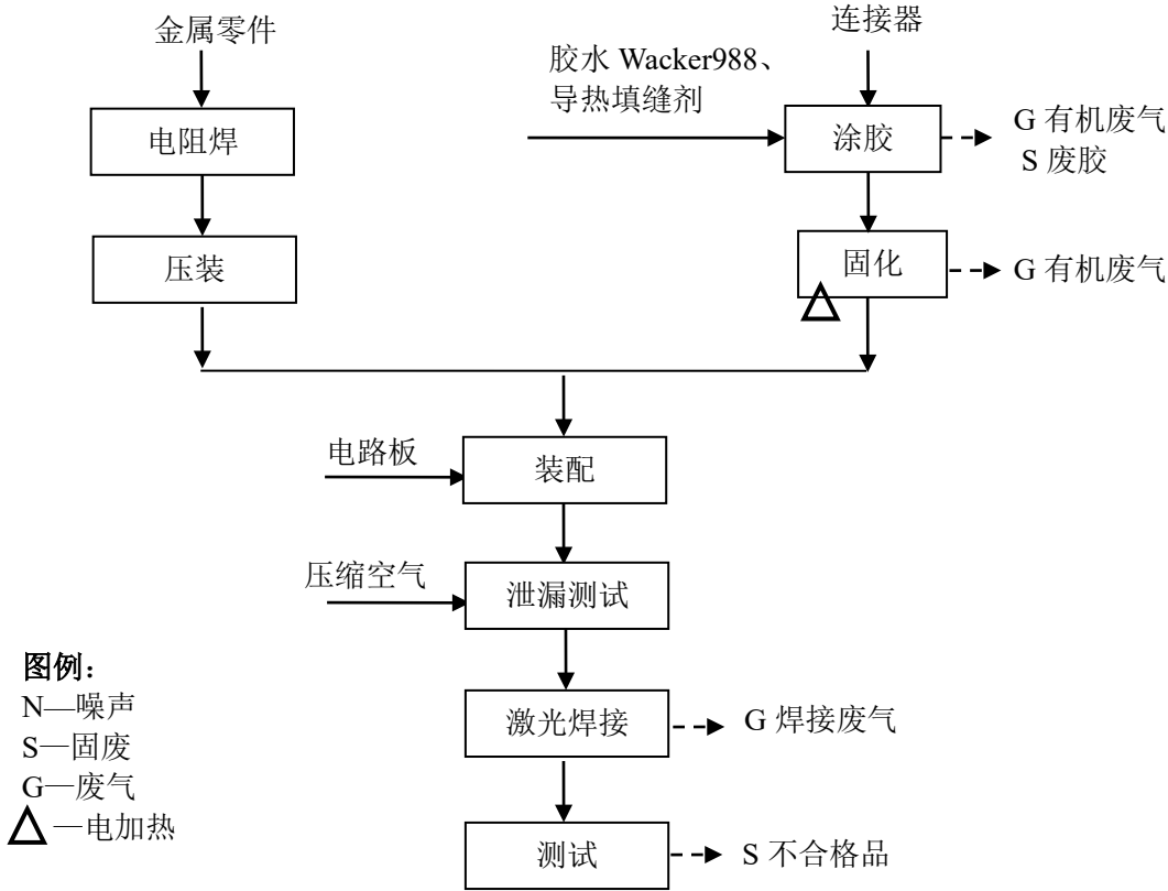
图2-11 TEF 实验室工艺流程图
