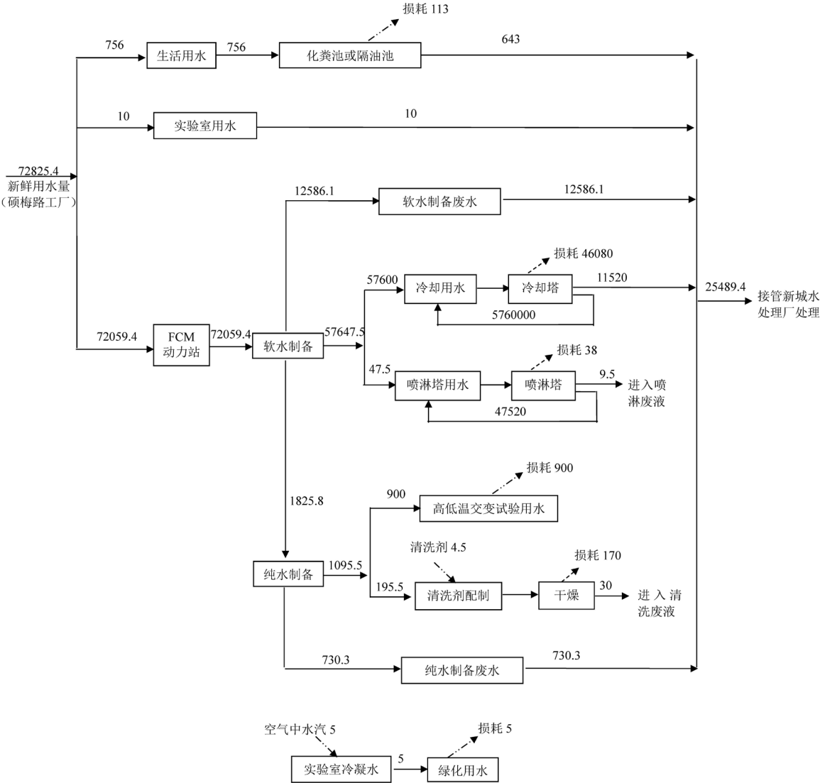
图2-1 本项目水（汽）平衡图 （单位：吨/年）
