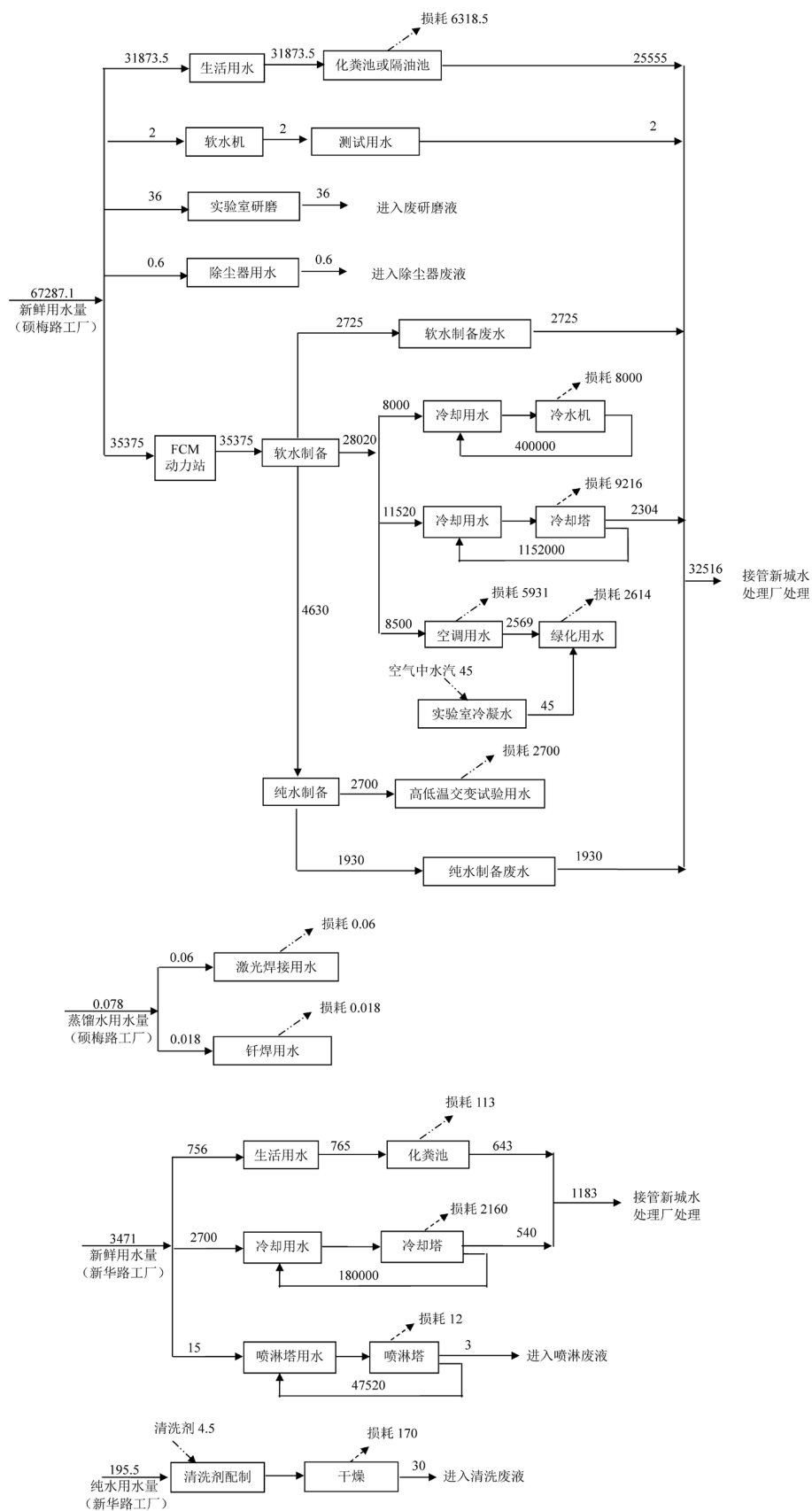
图2-13 现有项目水（汽）平衡图（单位：t/a）
