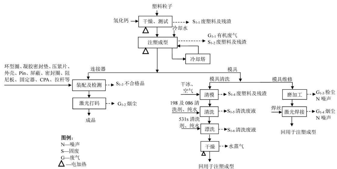
图2-12 高压连接器、低压连接器工艺流程图
