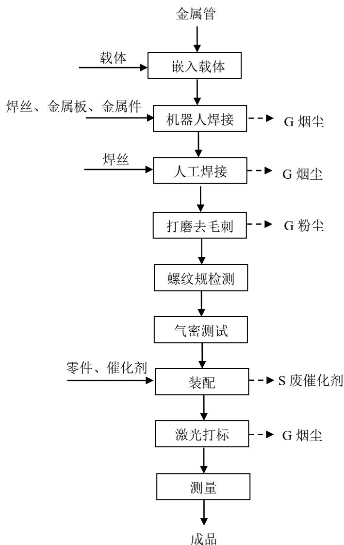
图2-7 ATS 生产工艺流程图
