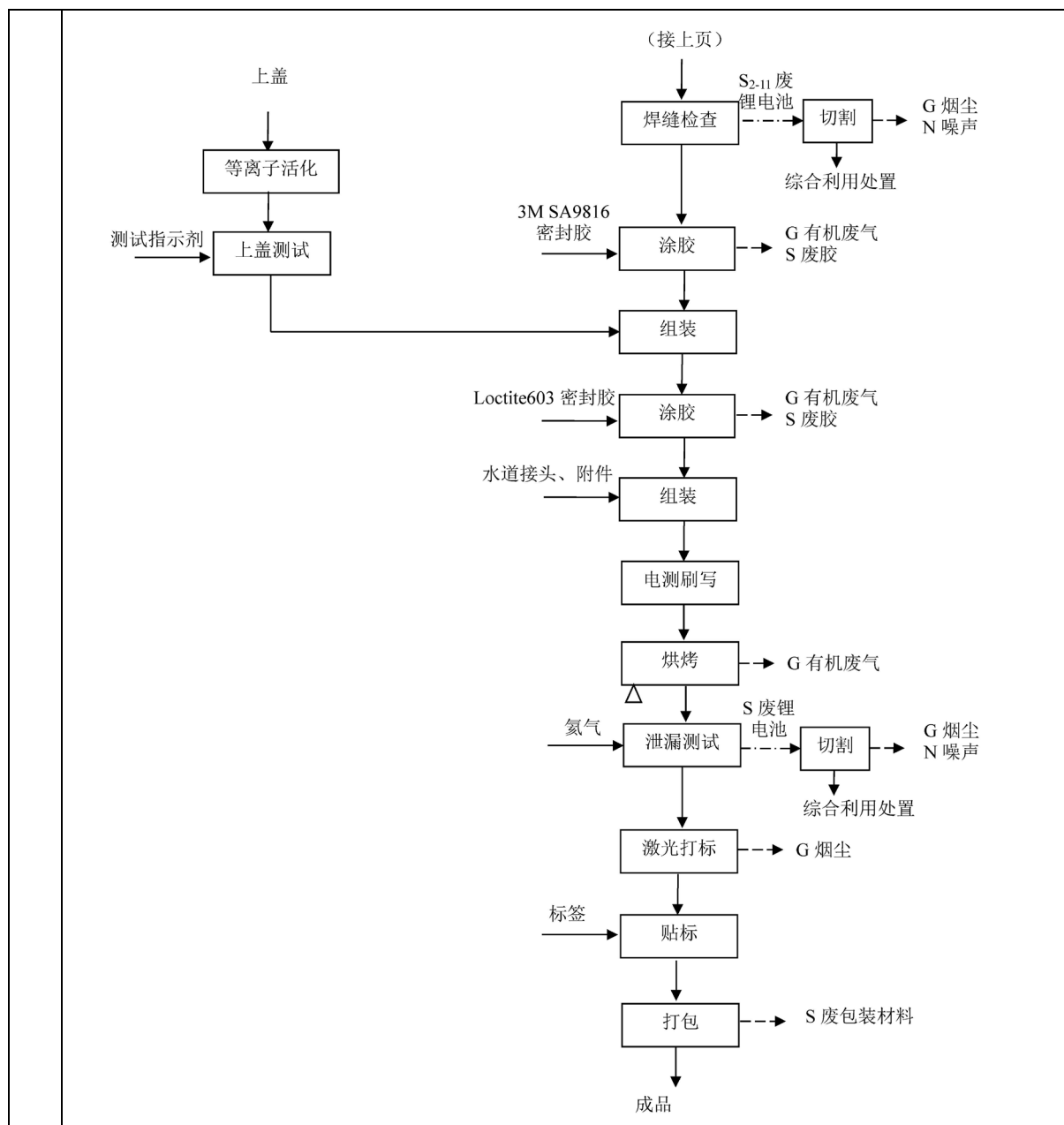
图2-10 48V2 代电池包工艺流程图
