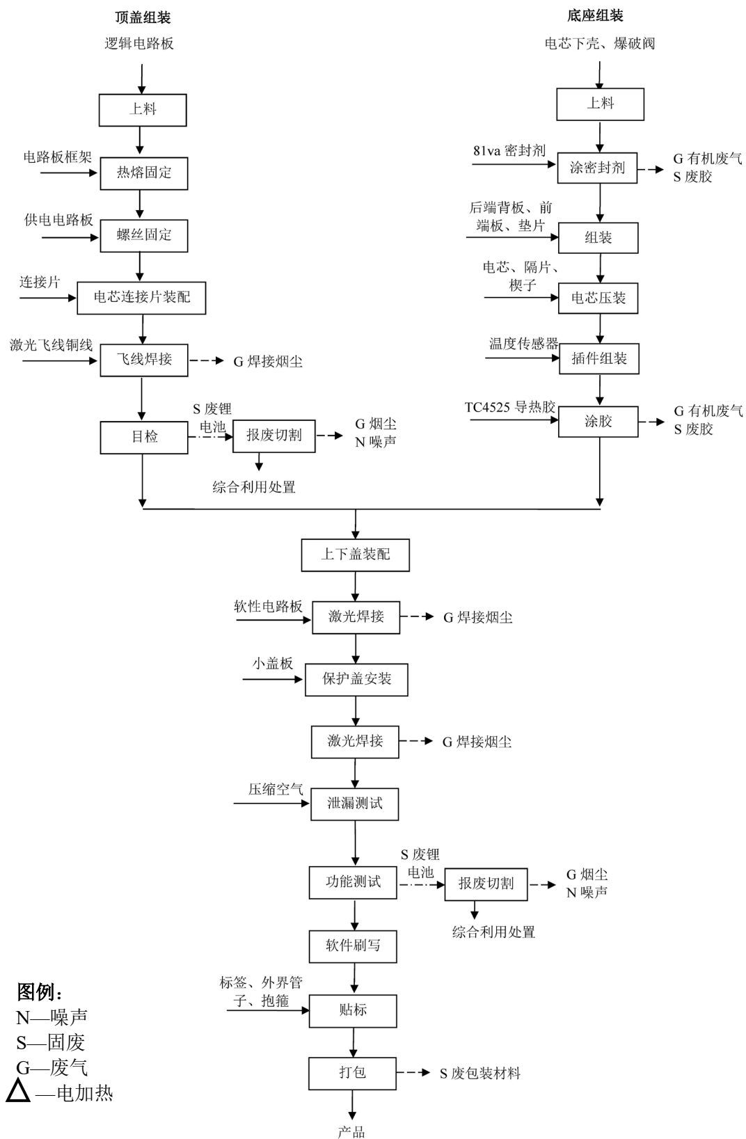
图2-9 48VLight 电池包工艺流程图
