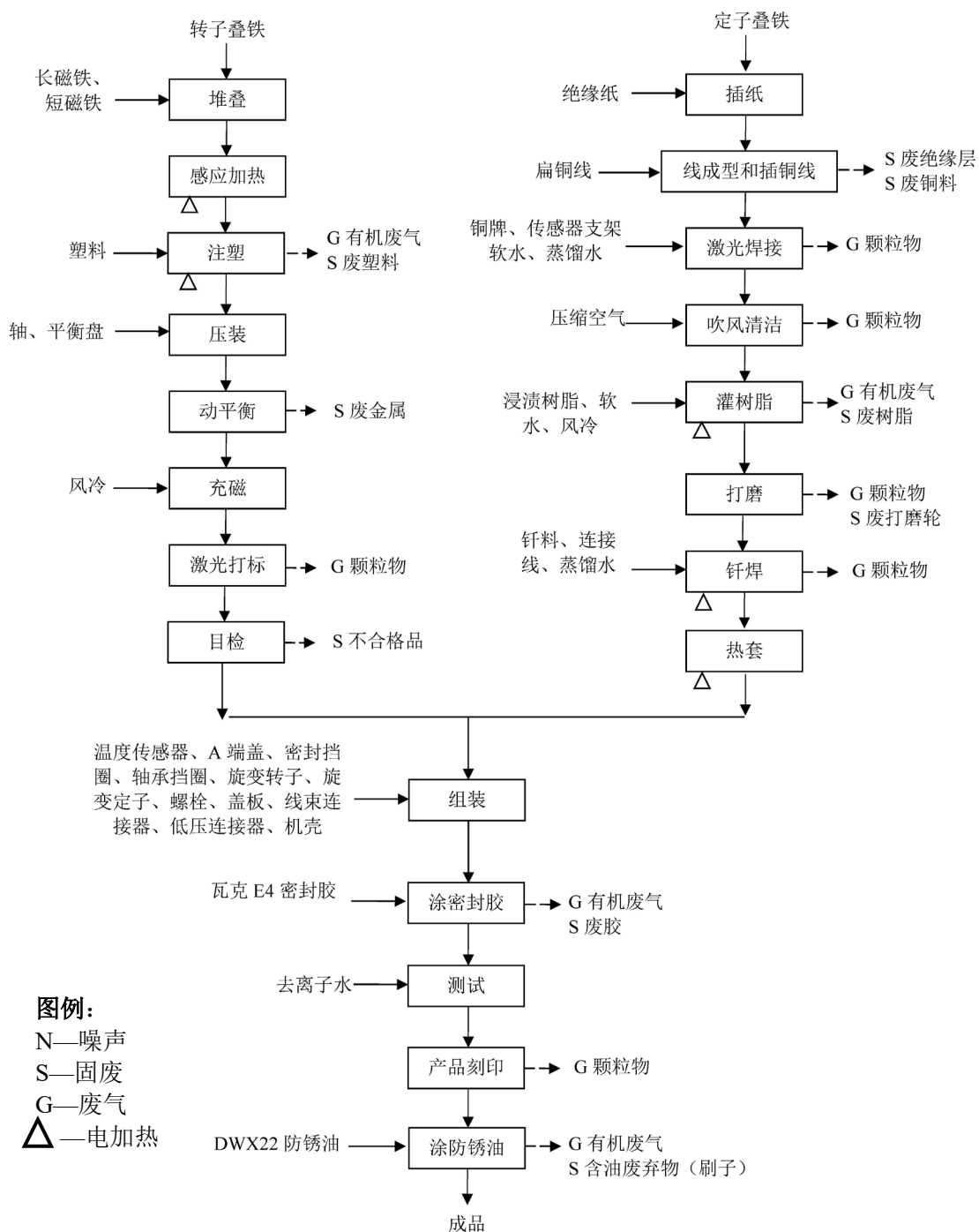
图2-8 SMG230 电机工艺流程图
