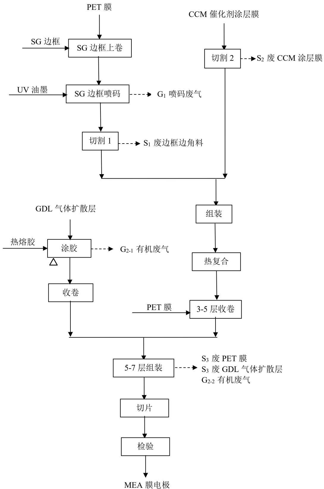
图 2-1 膜电极生产工艺流程图
