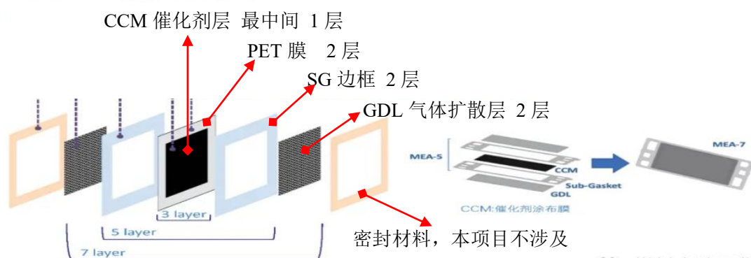
图 2-2 膜电极结构定义示意图
