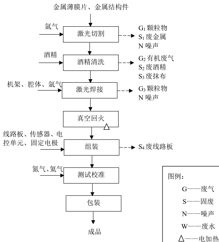
图 2-1 真空计生产工艺流程
