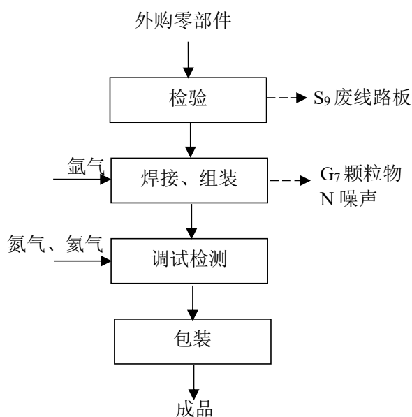
图 2-5 质谱仪生产工艺流程图
