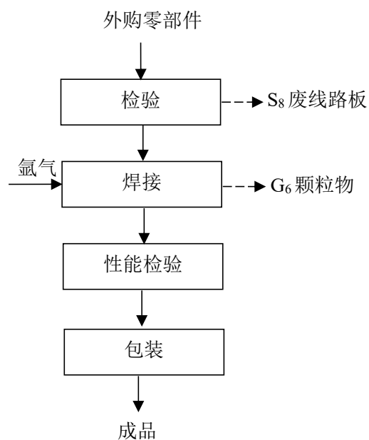
图 2-4 二次电源生产工艺流程图
