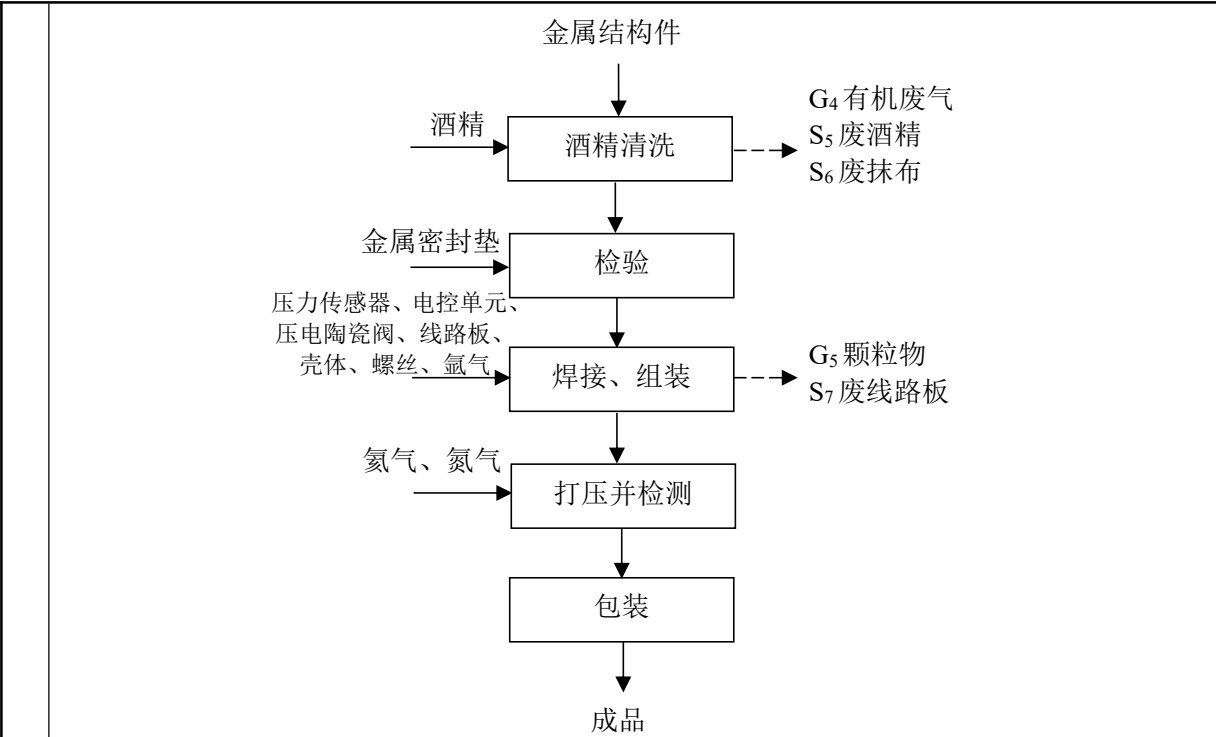
图 2-3 质量流量控制器生产工艺流程图
