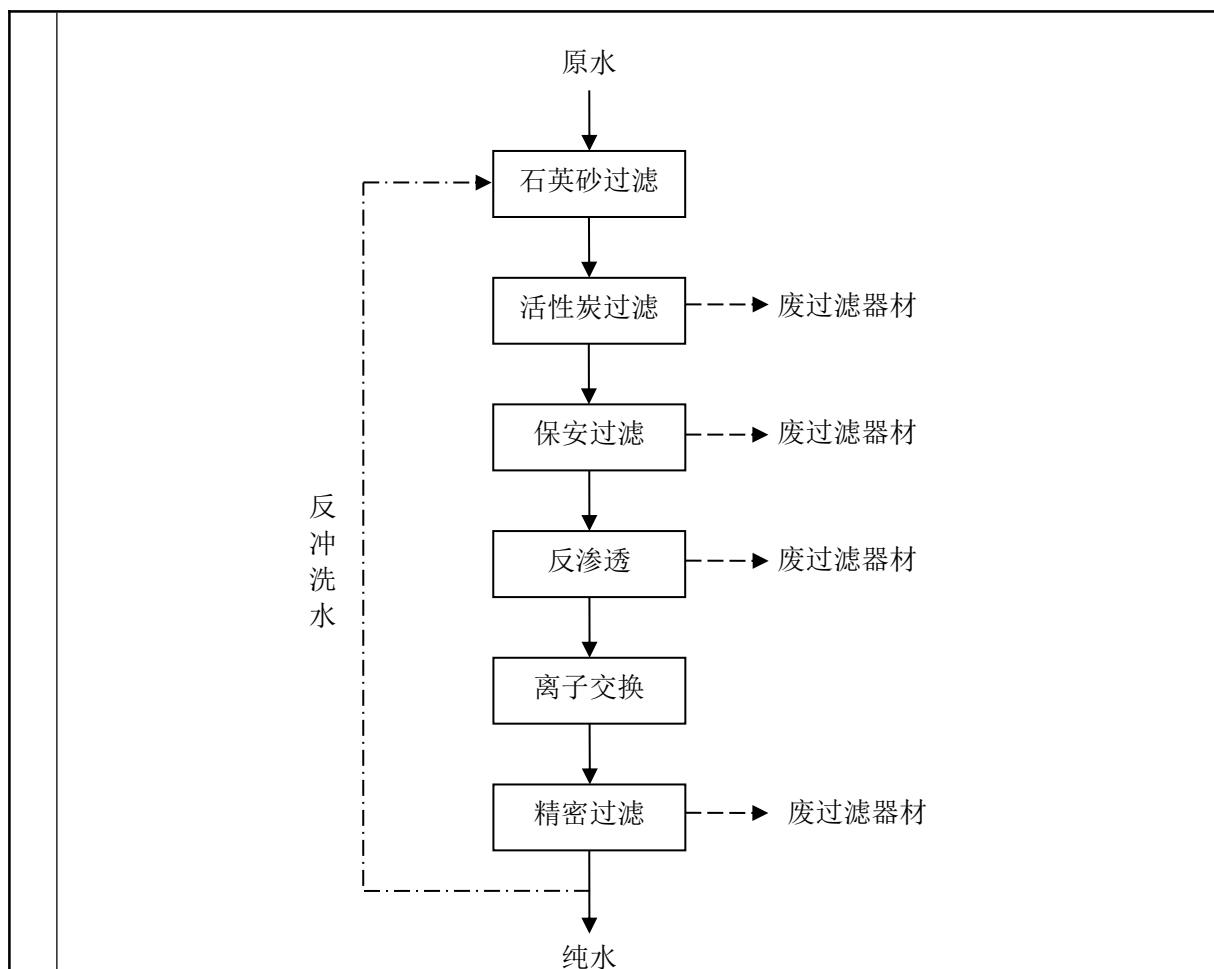
图 2-7 纯水制备工艺流程图
