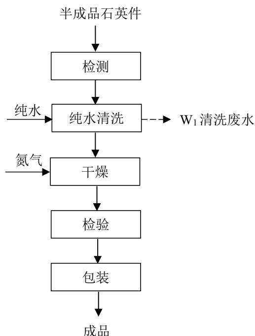
图 2-2 石英件生产工艺流程图
