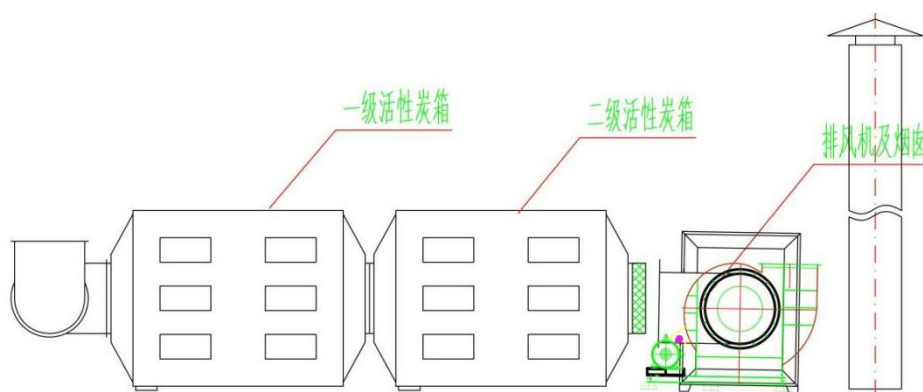
图 4-2 活性炭吸附装置内部结构图
