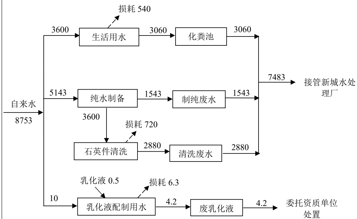
图 2-8 本项目水量平衡图 (单位: t/a)
